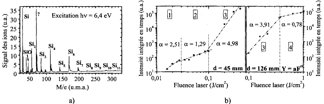
Figure 3. a) Spectre de masse typique des espèces éjectées au cours de l'irradiation des nano-agrégats de Si déposés. Fluence d'irradiation : 0,5 \text{ J/cm}^2 . b) Variation de l'intensité Y des ions \text{Si}^+ désorbés à partir des nano-agrégats en fonction de la fluence laser F (échelles logarithmiques). Deux distances cible – spectromètre de masse ont été utilisées: d = 45 \text{ mm} pour les plus faibles fluences ( 0,02\text{-}0,4 \text{ J/cm}^2 ), d = 126 \text{ mm} pour les plus grandes fluences ( 0,1\text{-}0,9 \text{ J/cm}^2 ).
